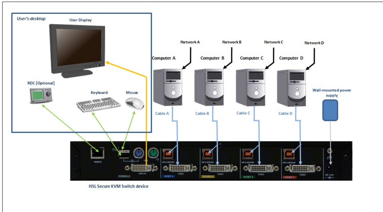
התקנת מוצר אופיינית – K204I
